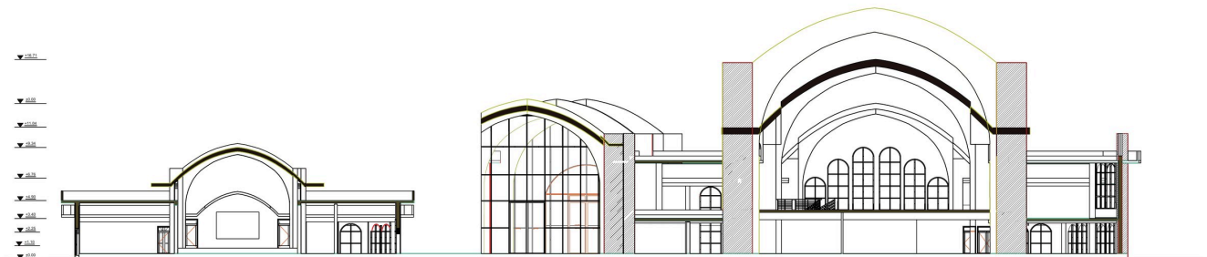
Schnitt 1/1 mit Spitzbogengewölbe über dem Saal. Zeichnung: Ahmad Milad Toryalai
